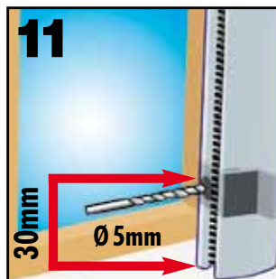
11/12 Percez les glissières et le mur au Ø 5 mm en utilisant le gabarit.
