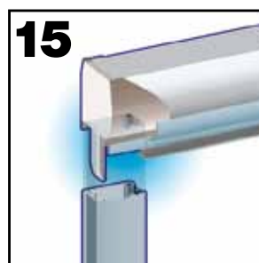
15 Réunir l'ensemble coffre et glissières. 16 Visser les glissières pour une fixation définitive.
